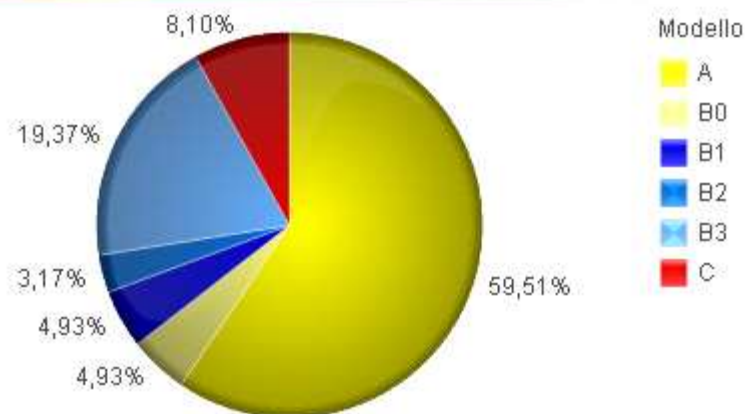
% modelli compilati
